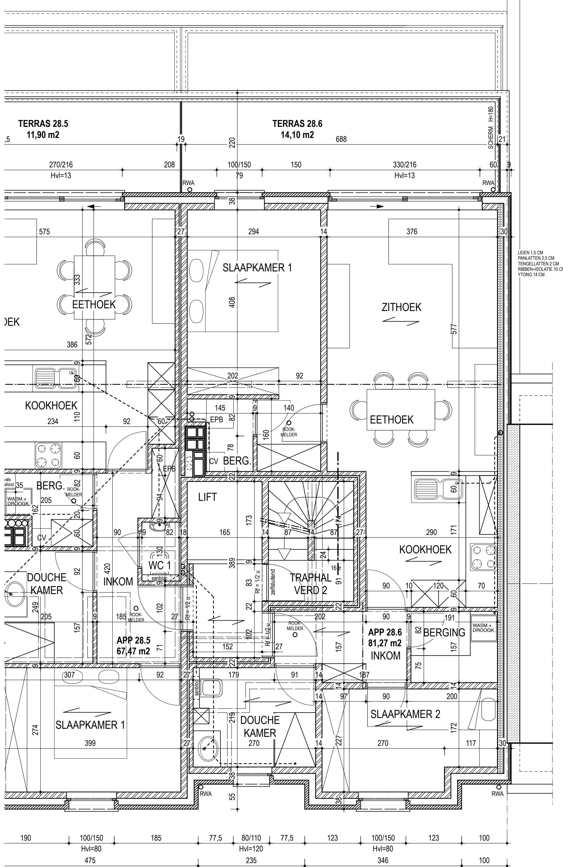
verdieping 2 schaal 1/50 1 m hoogte binnendeuren = 217
