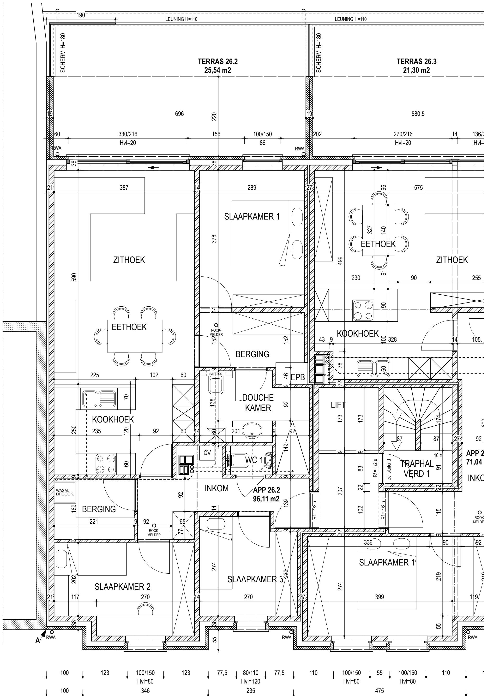
verdieping 1 schaal 1/50 1 m hoogte binnendeuren = 217
